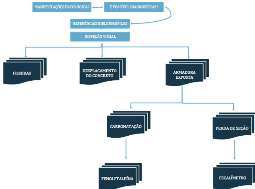
Figura 2 - Fluxograma da análise de corrosão em estruturas
